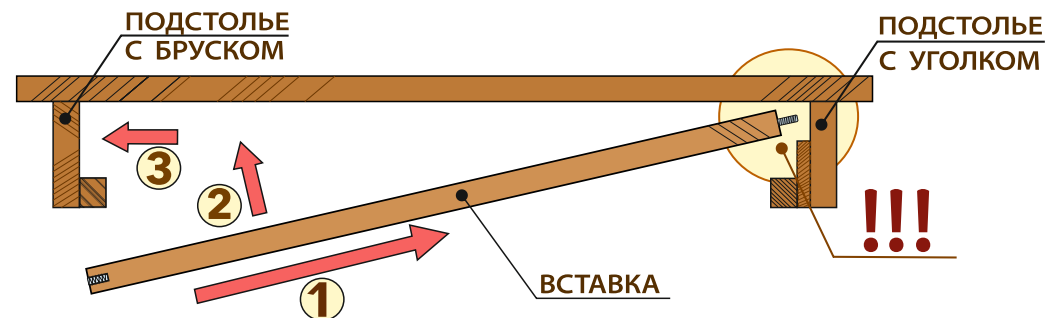
РИС. 2 ВИД СТОЛА СБОКУ
